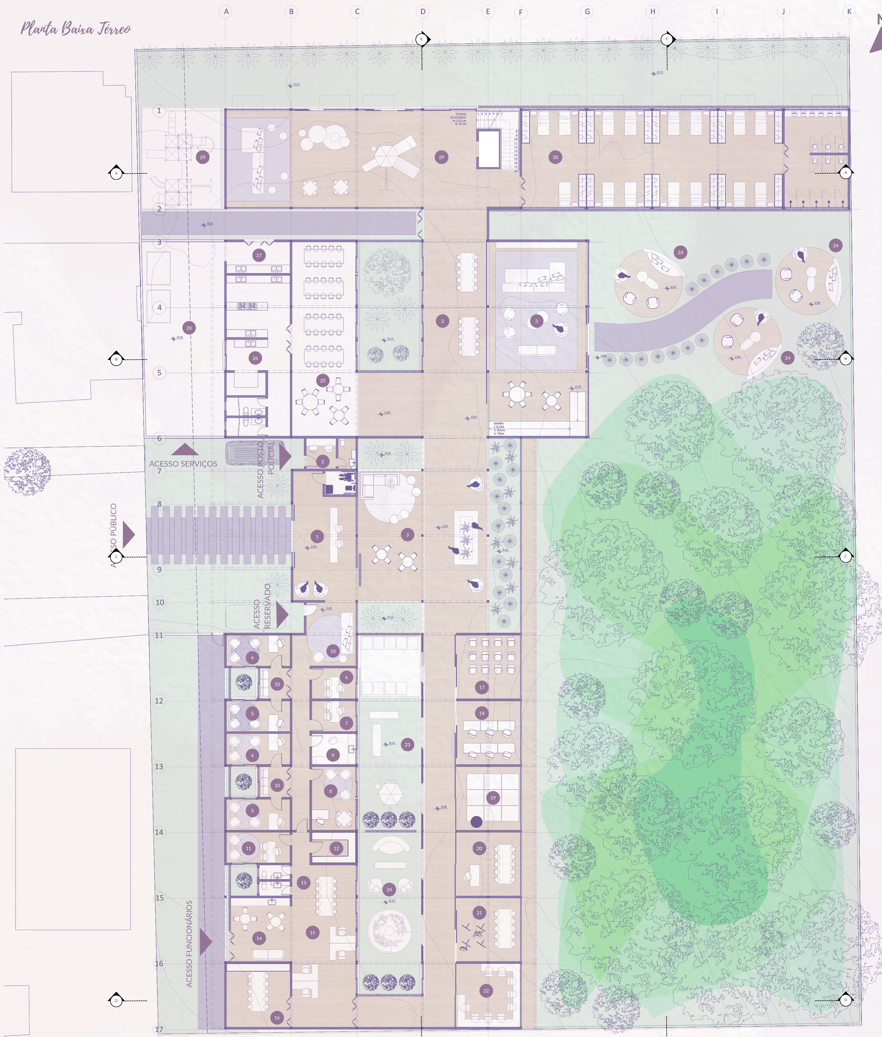
PLANTA BAIXA TÉRREO
