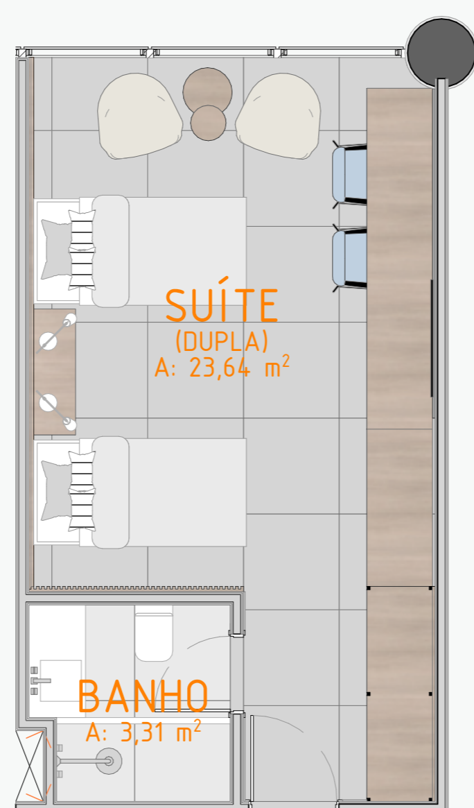
PLANTA BAIXA SUÍTE DUPLA 4º PAVIMENTO - 6 UNIDADES ESC.: 1/50
