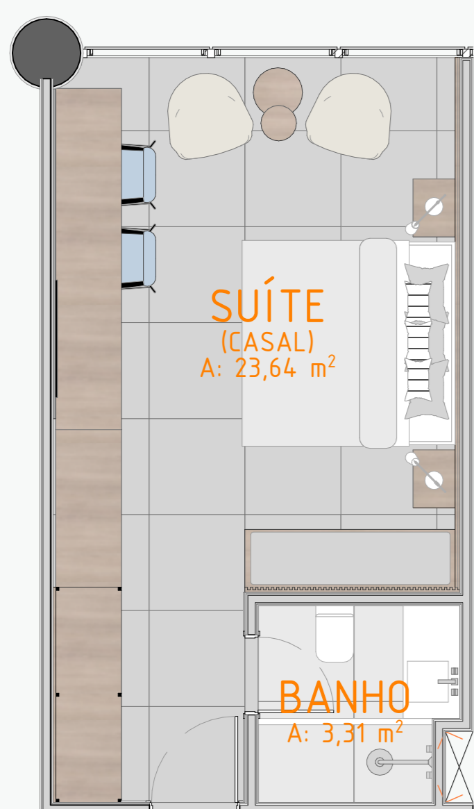
PLANTA BAIXA SUÍTE CASAL 3º PAVIMENTO - 6 UNIDADES ESC.: 1/50
