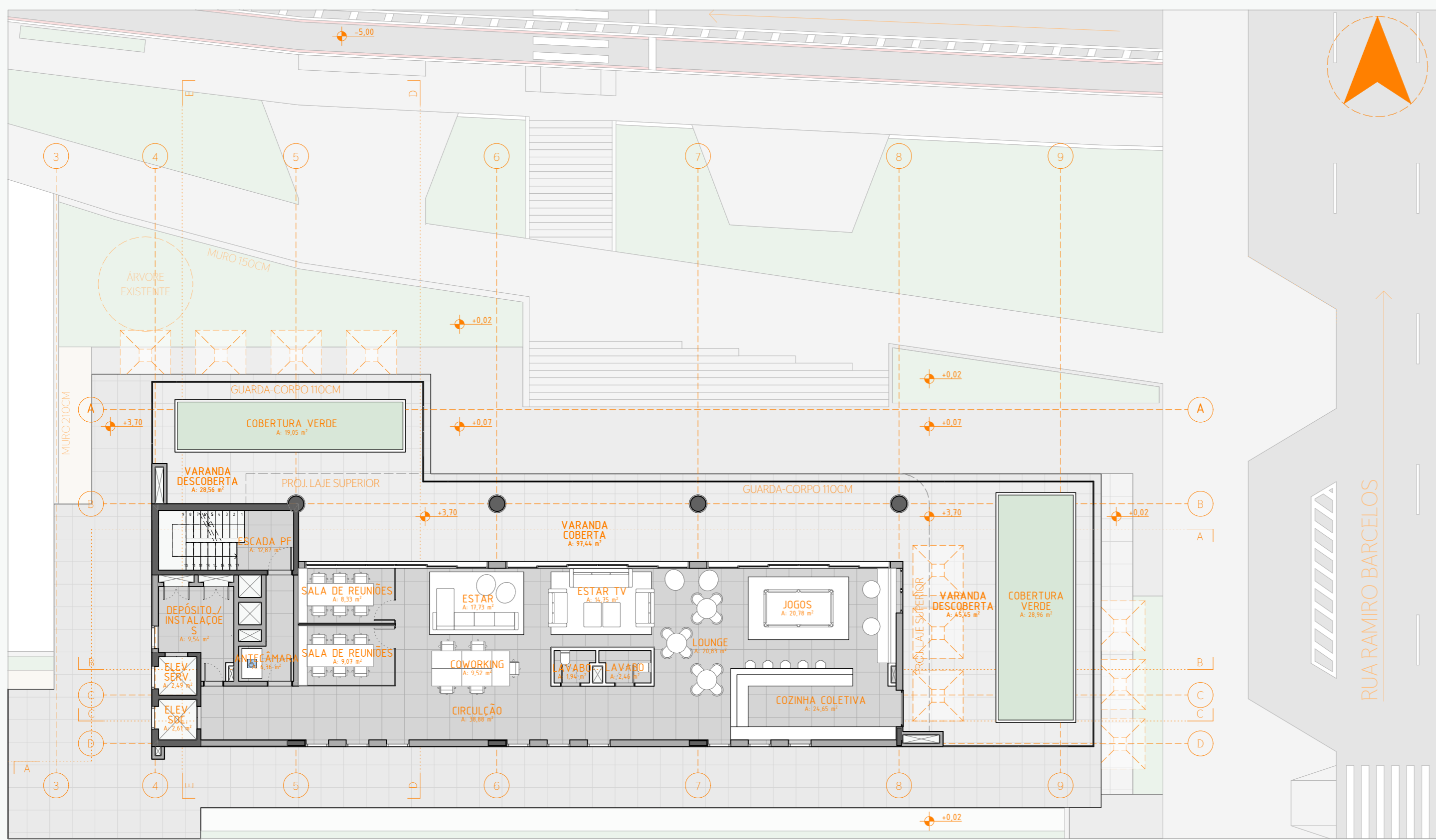
PLANTA BAIXA PAVIMENTO LAZER (2º) - ESC: 1/150 NÍVEIS: +3,70M
