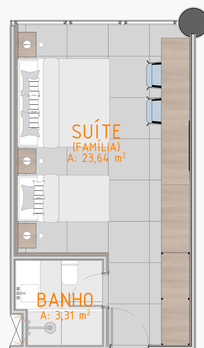
PLANTA BAIXA SUÍTE FAMÍLIA 5º PAVIMENTO - 6 UNIDADES ESC.: 1/50
