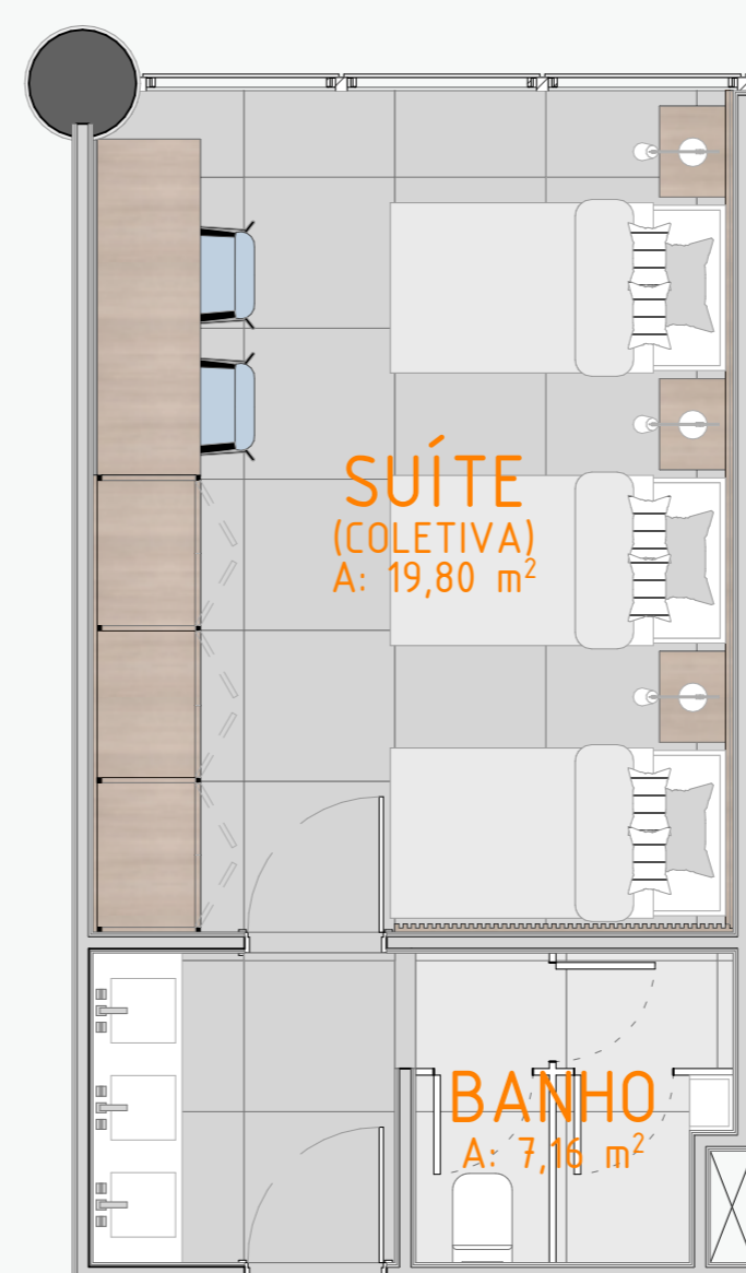
PLANTA BAIXA SUÍTE COLETIVA 6º E 7º PAVIMENTO - 12 UNIDADES ESC.: 1/50
