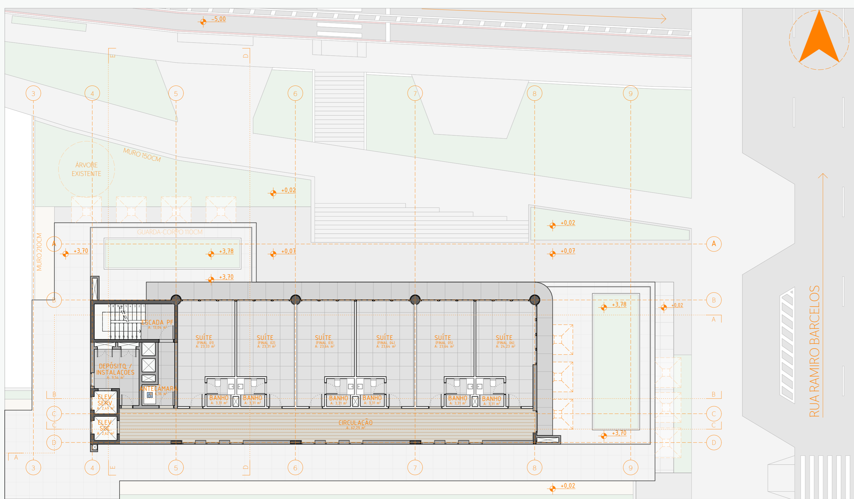
PLANTA BAIXA TIPO A - ESC: 1/150 NÍVEIS: +6,70M, 9,70M E 12,70M SUÍTES: COLETIVA
