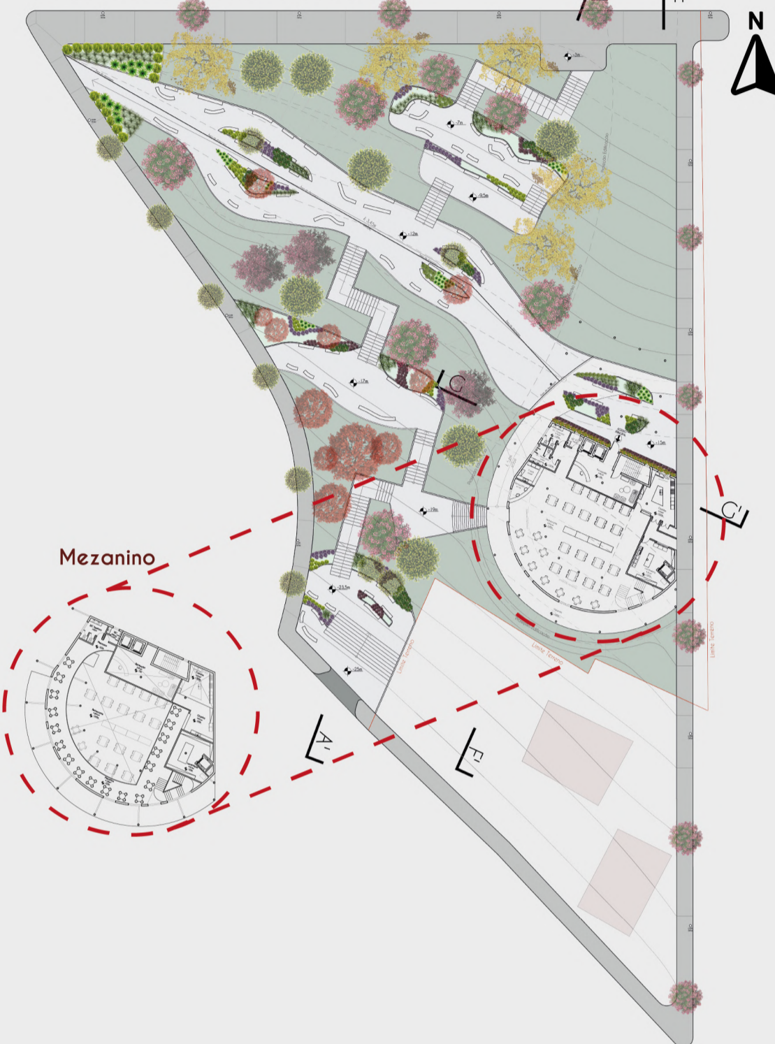
Planta Baixa Térreo
