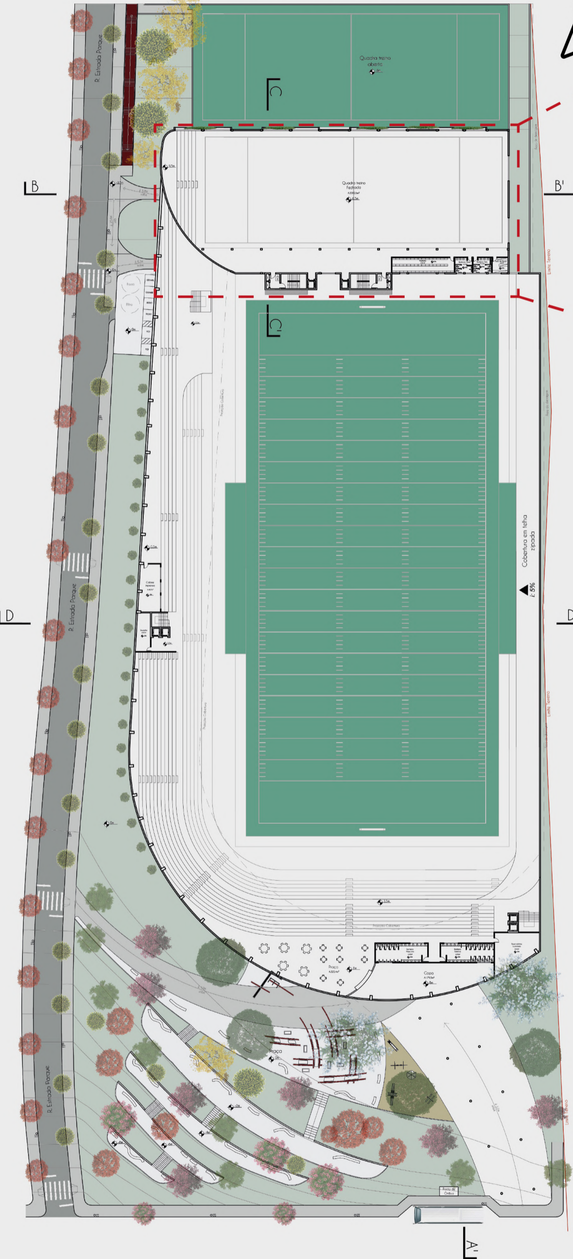
Planta Baixa 2º Pavimento
