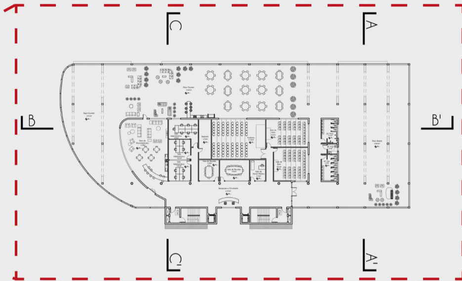
Planta Baixa 3º Pavimento
