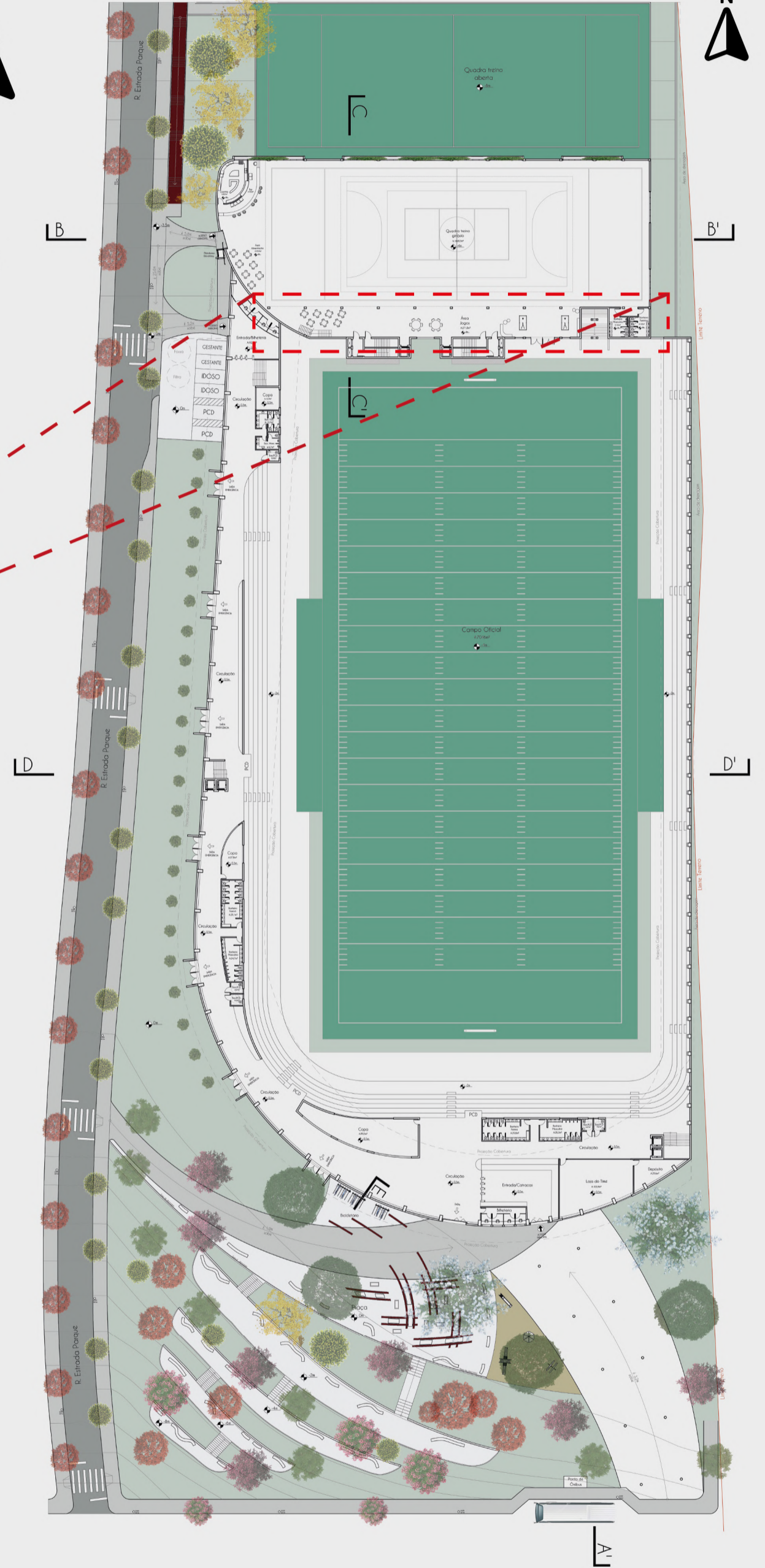
Planta Baixa Térreo
