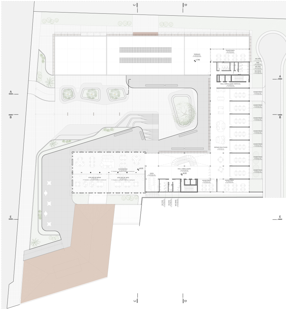
PLANTA BAIXA TERCEIRO PAVIMENTO Escala 1/200
