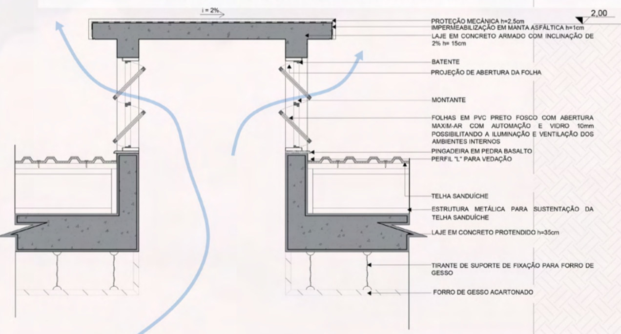
DETALHAMENTO VENTILAÇÃO CHAMINÉ
