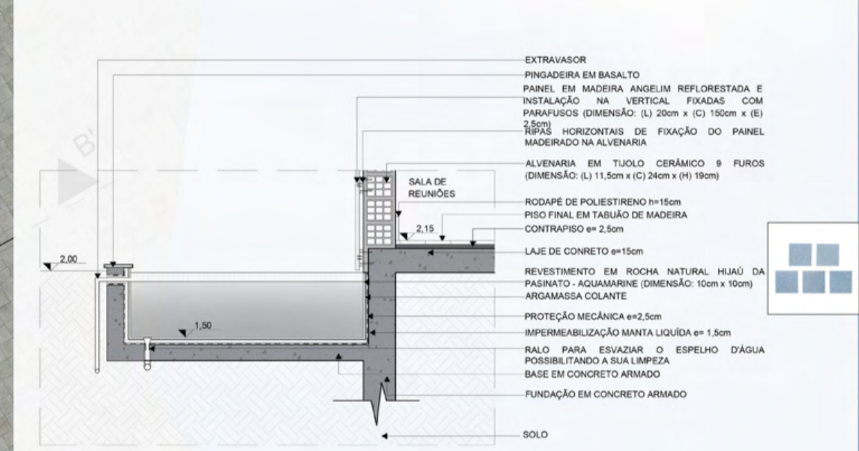
DETALHAMENTO DOS ESPELHOS D'ÁGUA
