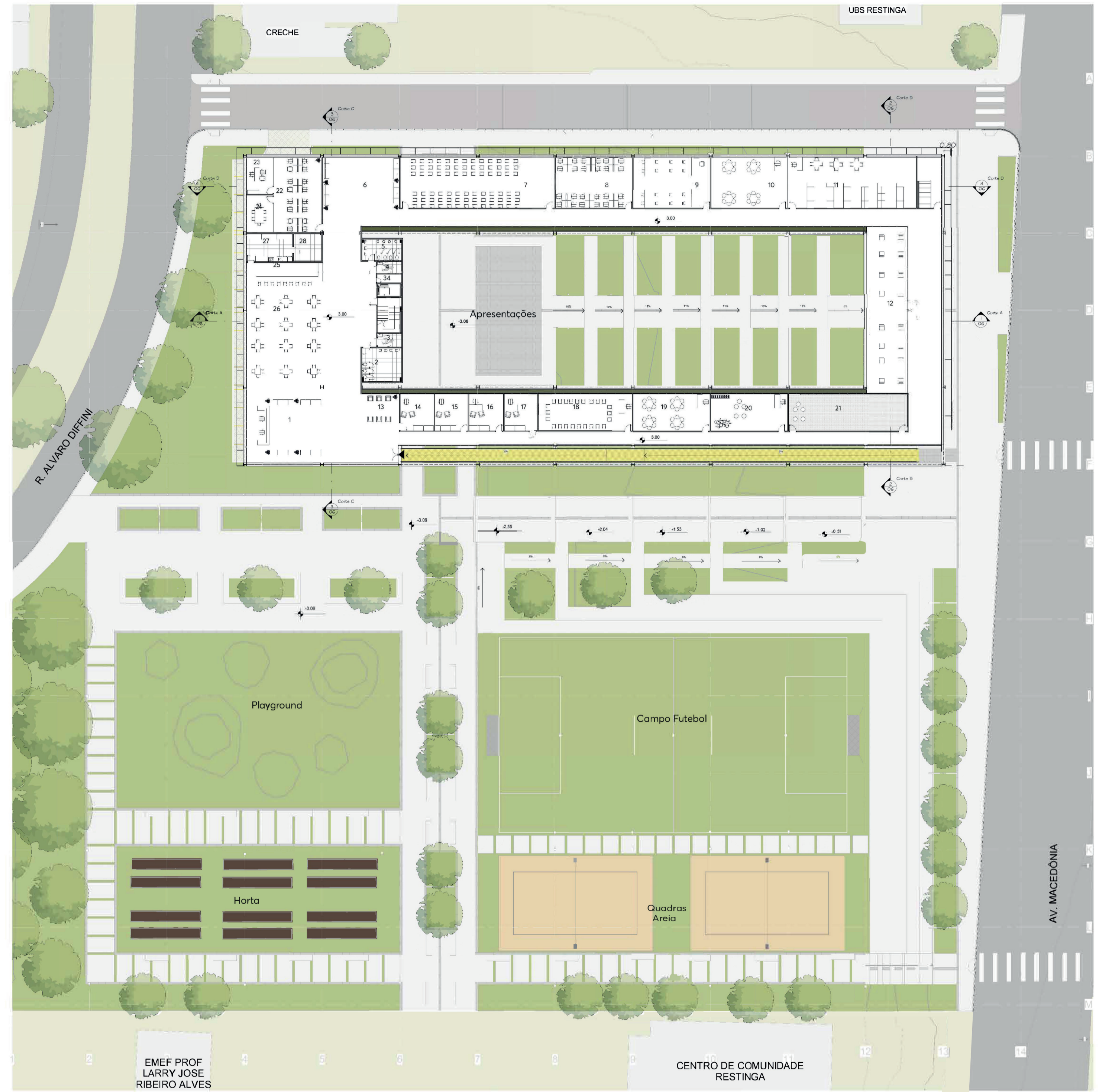
Térreo Planta Baixa 1/500
