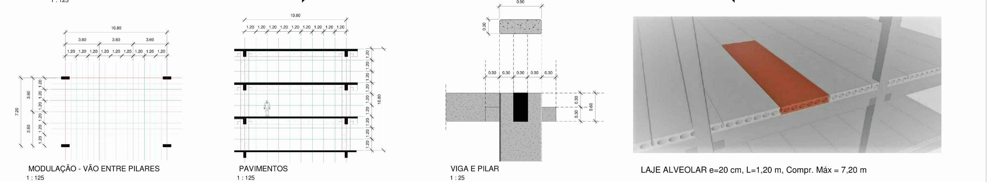
2º PAVIMENTO 1:125
