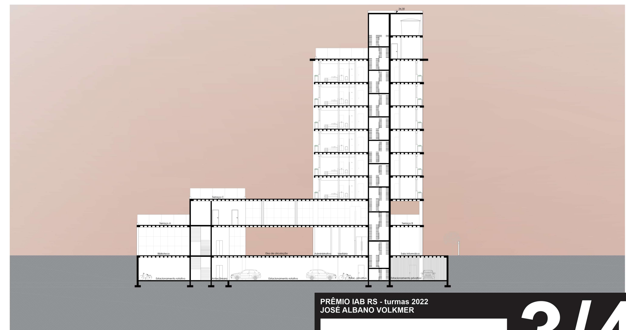
CORTE CC esc: 1/250
