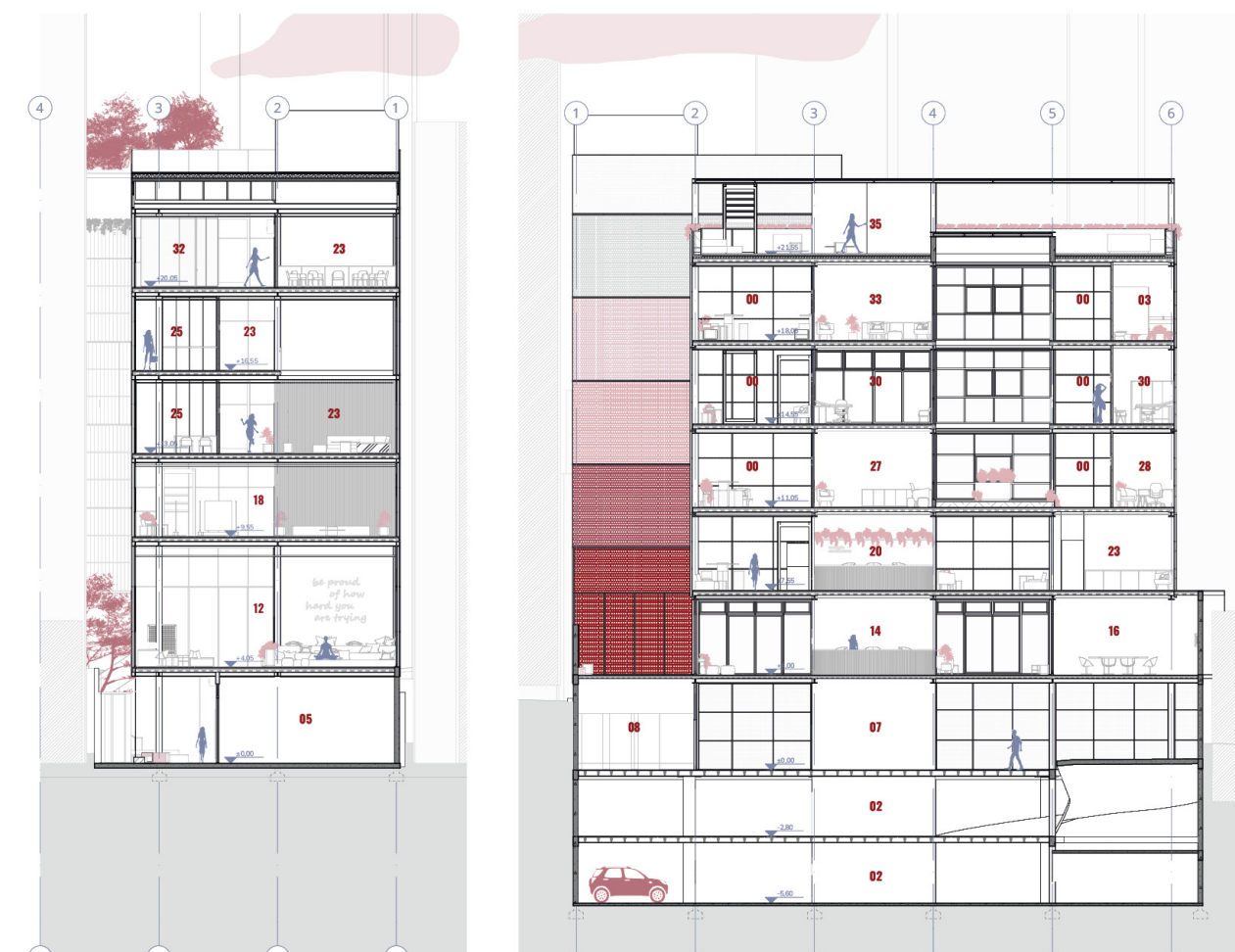
corte bb
