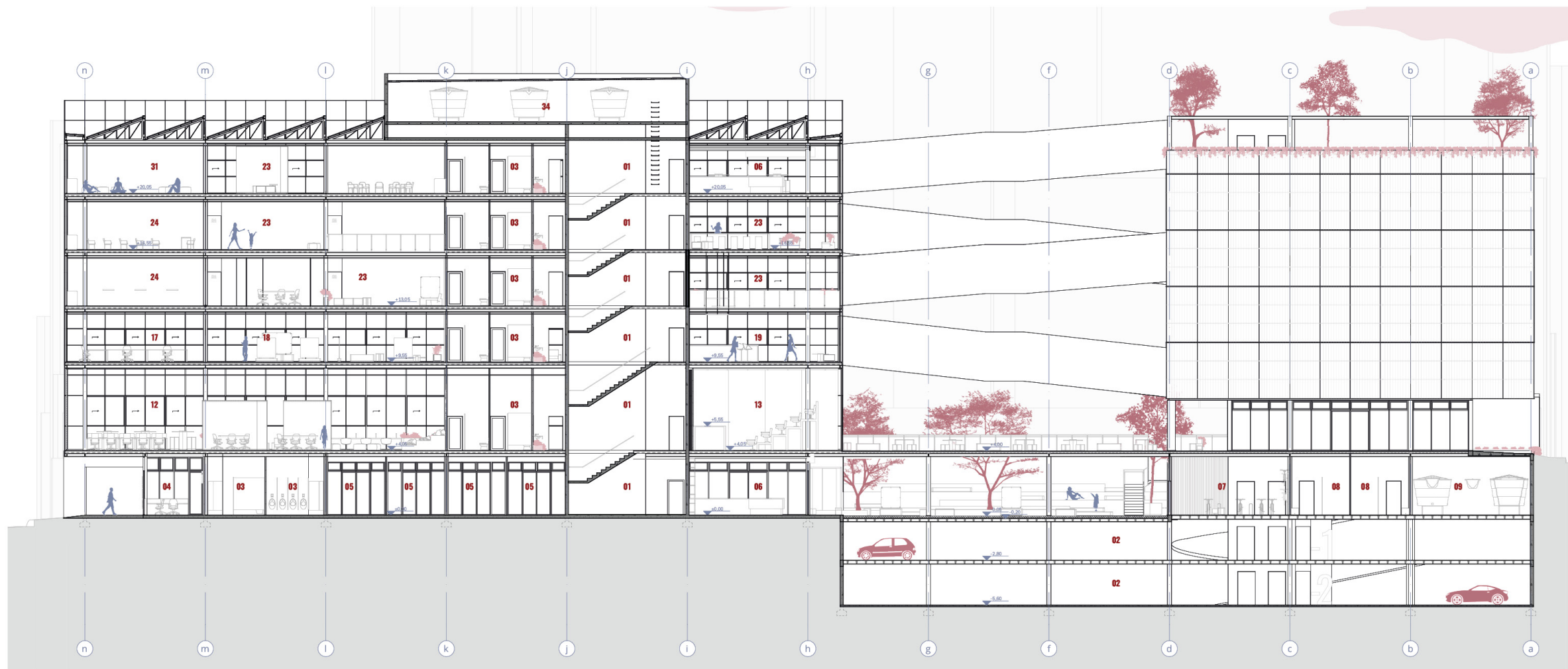
corte cc
