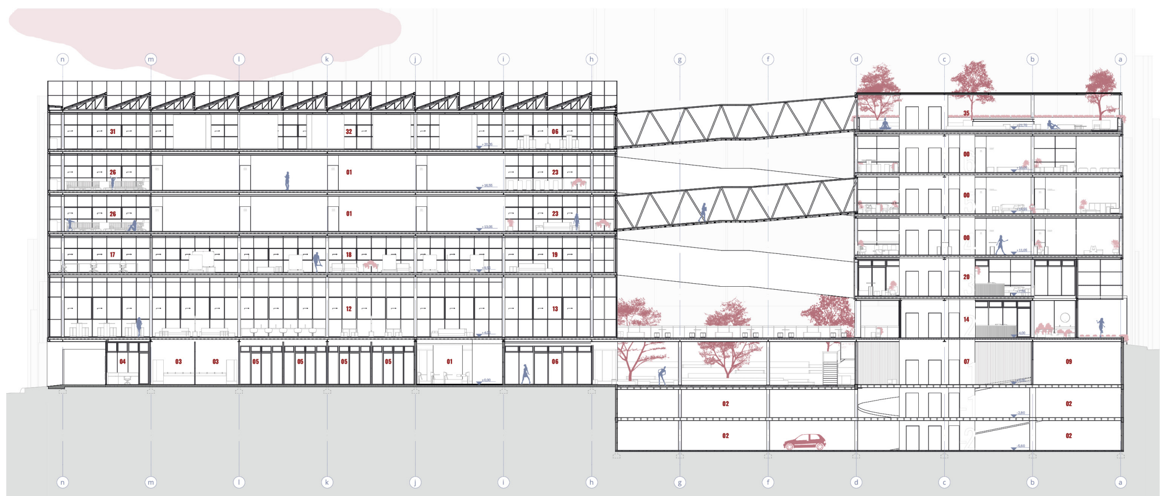
corte bb
