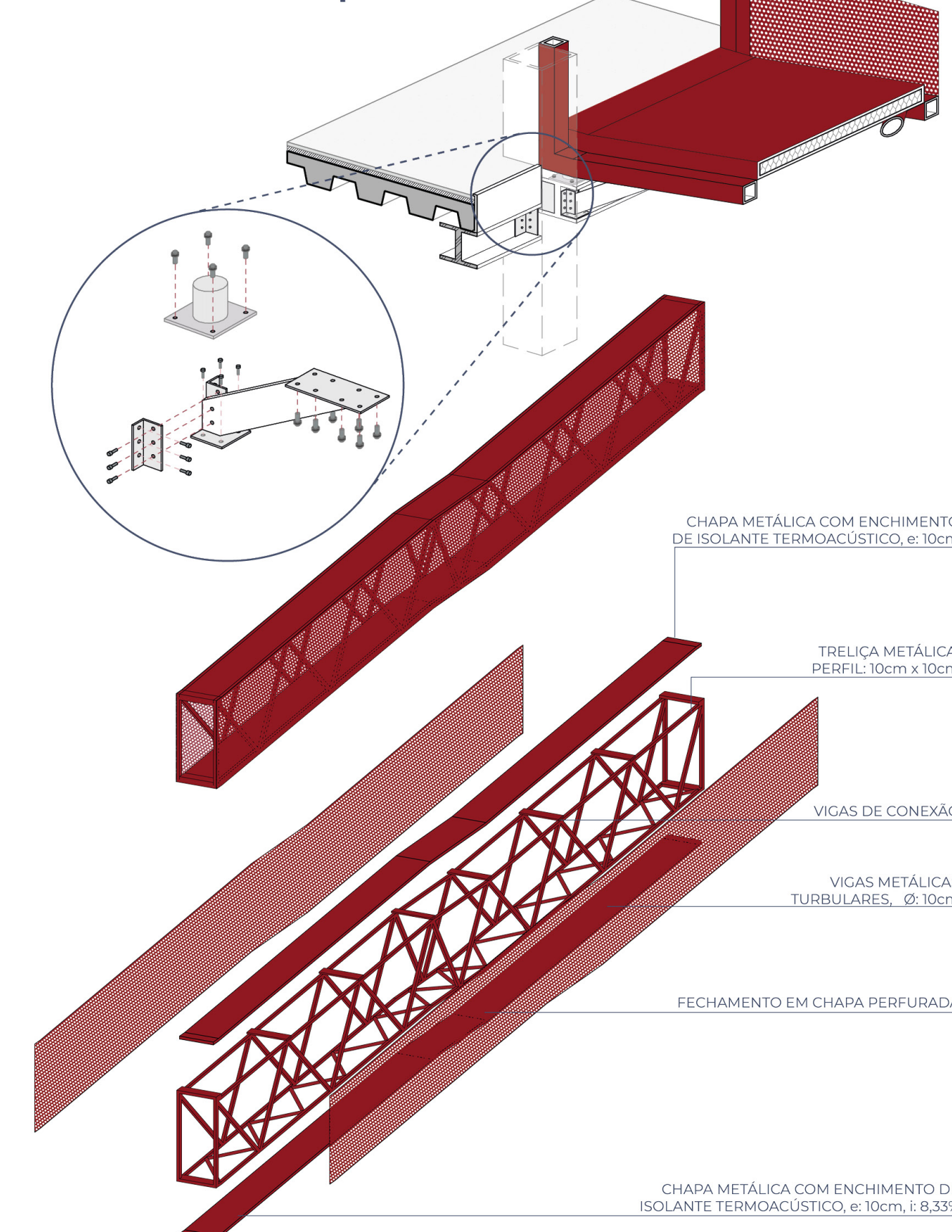
detalhamento rampa
