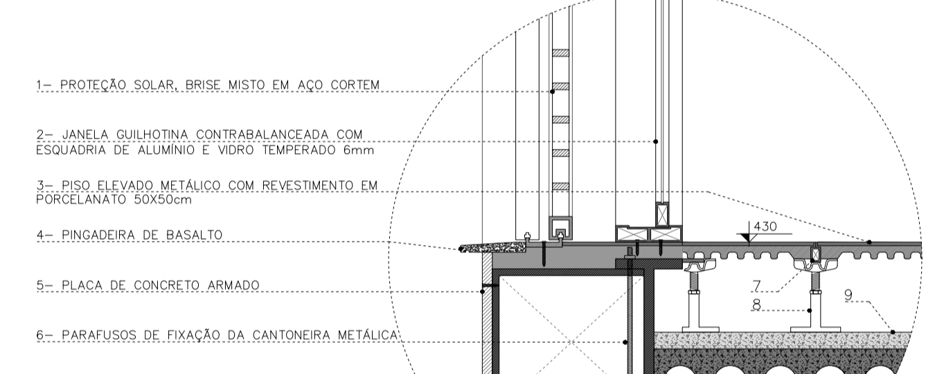
DETALHAMENTO 2: FECHAMENTOS JUNTO AO PISO ESCALA 1/10
