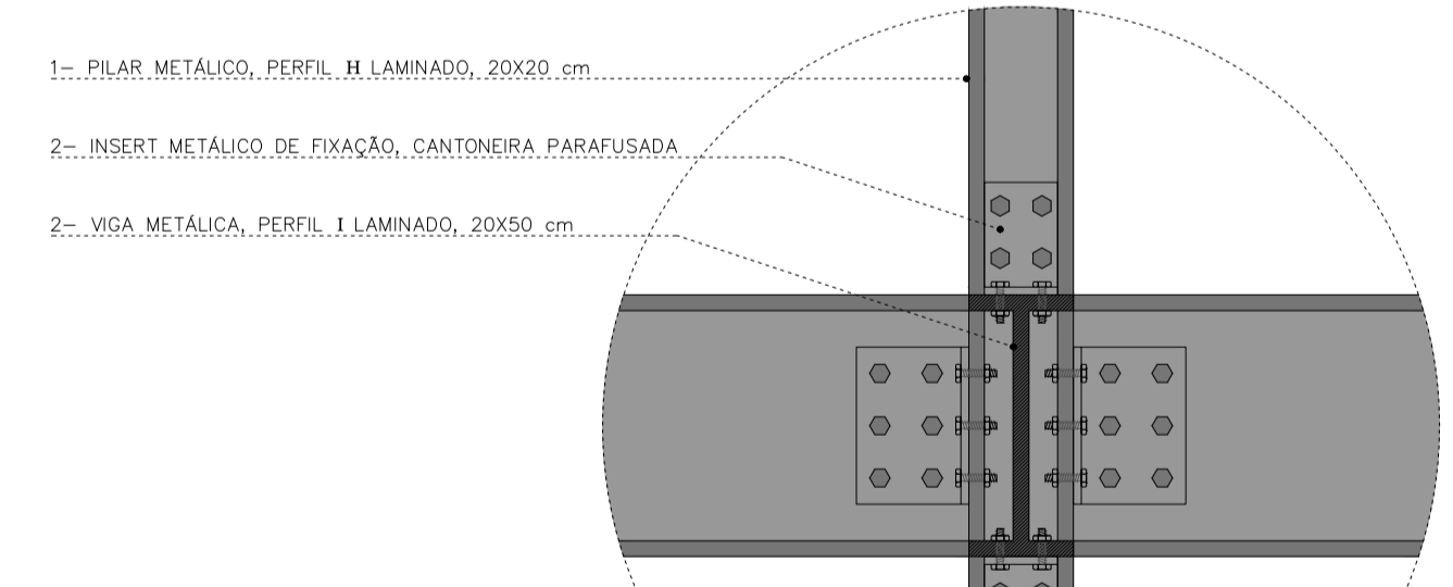
DETALHAMENTO 3: VIGA AÉREA DE BORDA ESCALA 1/10
