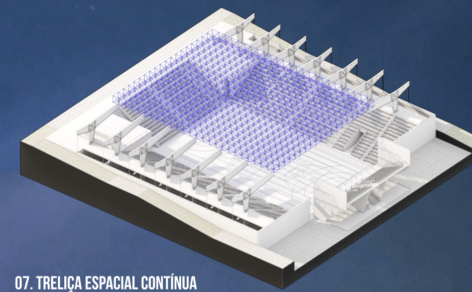
07. TRELIÇA ESPACIAL CONTÍNUA MÓD. 2.00X2.10M
