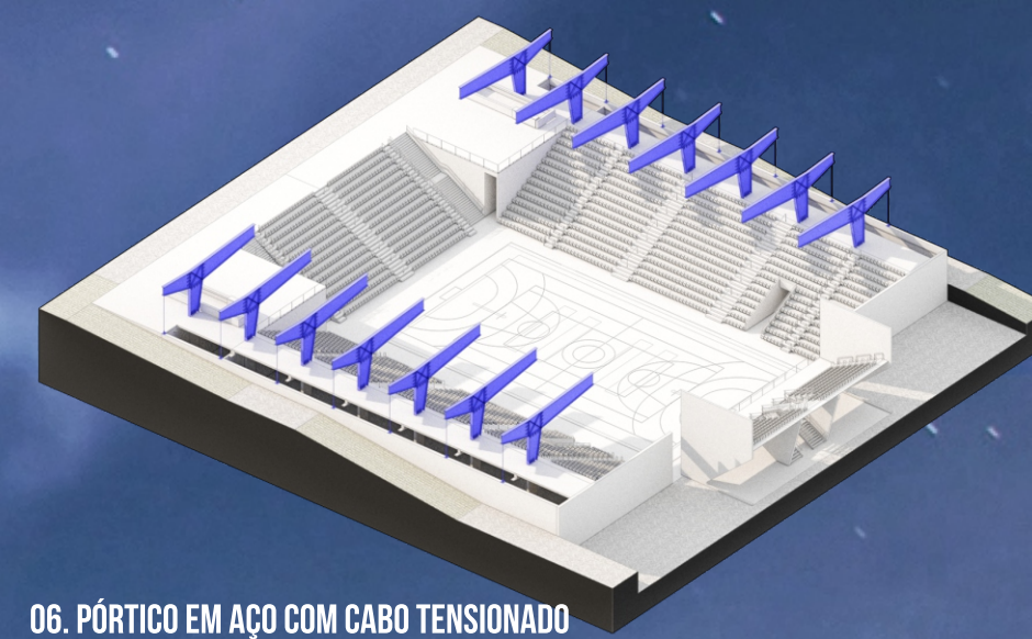
06. PÓRTICO EM AÇO COM CABO TENSIONADO MÓD. 8.40M ENTRE EIXOS
