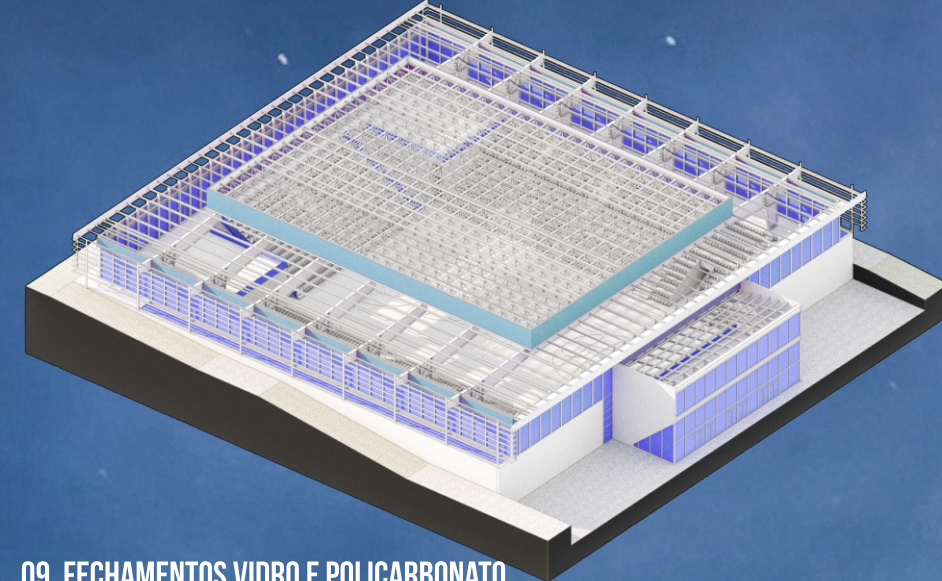
09. FECHAMENTOS VIDRO E POLICARBONATO
